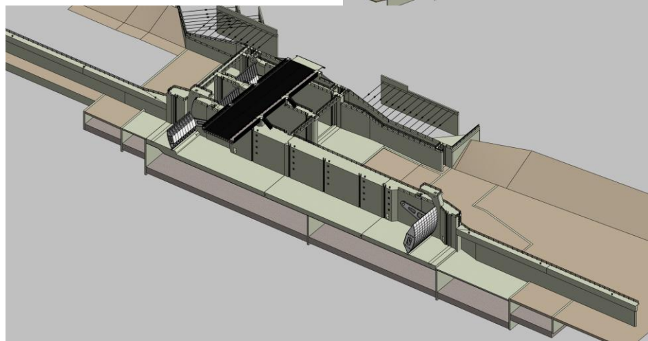
Hajózsilip hosszmetsete
