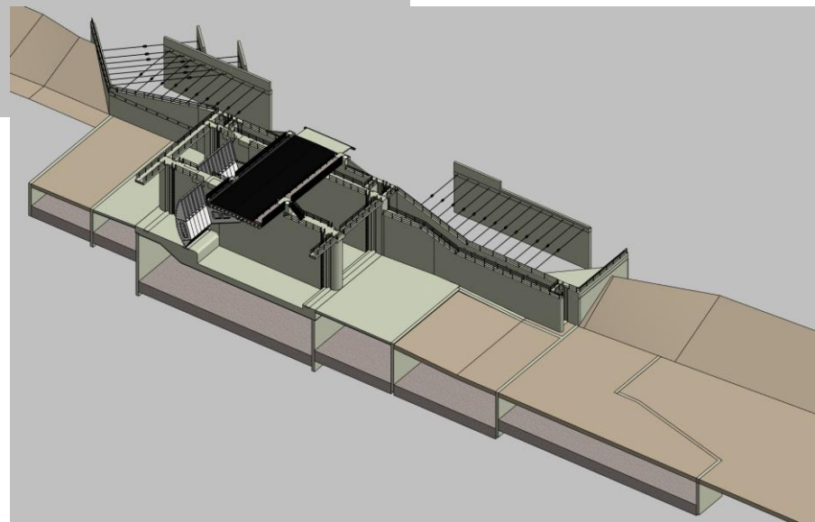
Leeresztőzsilip metszete
