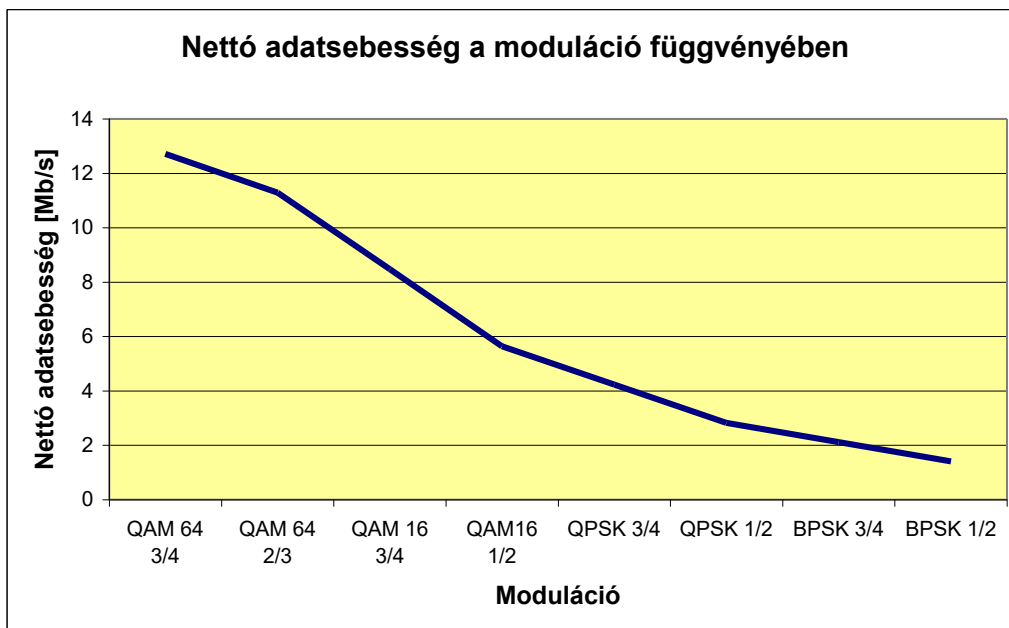
29. ábra. Egy P-MP rendszer nettó adatsebessége a moduláció függvényében
