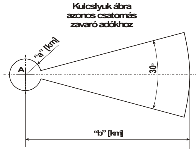
19. ábra. Kulcslyuk ábra azonos csatornás zavaró adókhöz
