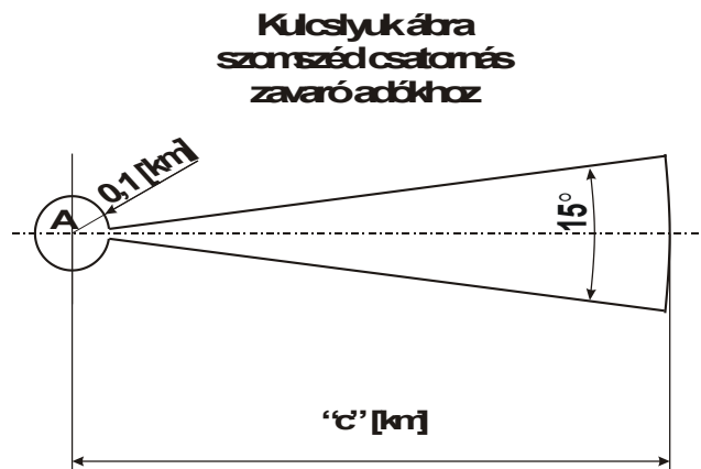
20. ábra. Kulcslyuk ábra szomszéd csatornás zavaró adókhöz
