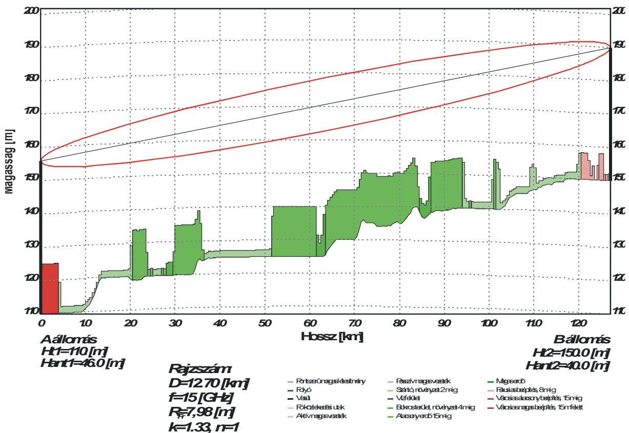
11. ábra. Terepmetszet
