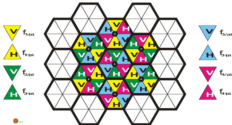
33. ábra. Hat szektoros cellákból álló P-MP rendszer
