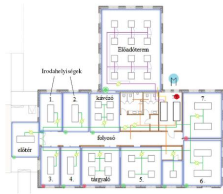
27.15. ábra: SRI2 - Alaprajz
