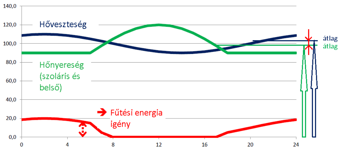
3.3. ábra. Veszteségek és nyereségek időbeni változása egy nap során (alacsony energiaigényű épület) (Dick van Dijk BUILD UP Webinar seriesWebinar 4: EPB standards hourly vs monthly methods 26 May 2020)
