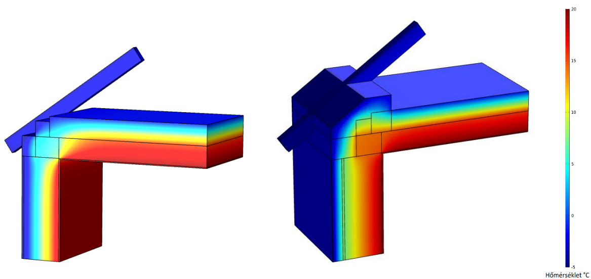
20.10. ábra. Hőszigetetlen 37,5 cm vastagságú pórusbeton falazóblokkból épített falszerkezet és 20 cm szálas hőszigeteléssel ellátott pórusbeton pallófödém hőszigetetlen talpszelemen kialakítással (balra) és 10 cm külső oldali hőszigeteléssel ellátott 37,5 cm vastagságú nagyszilárdságú pórusbeton falazat 20 cm szálas szigeteléssel ellátott pórusbeton pallófödémrel és körbehőszigetelt talpszelemennel (jobbra)
